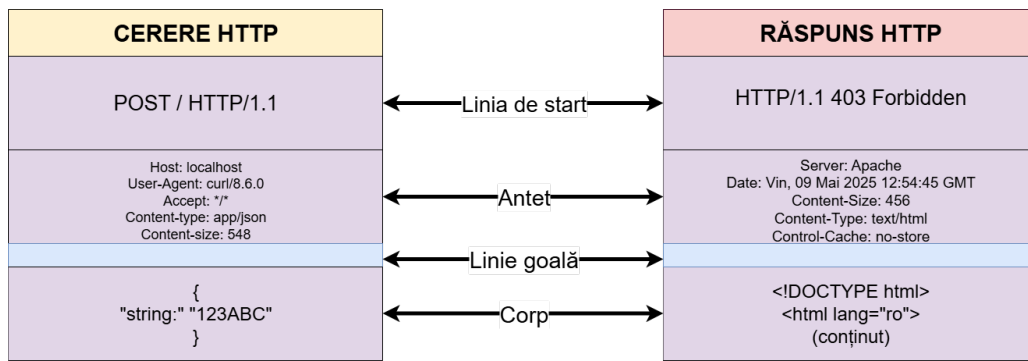
Figura 2.12: Răspuns HTTP
