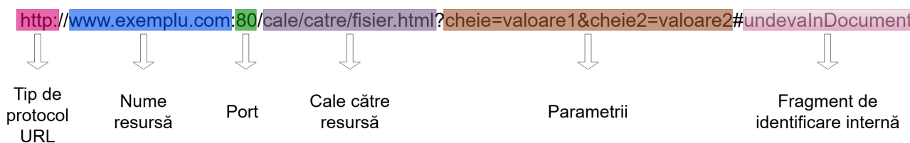
Figura 2.2: Componentele URL-ului
